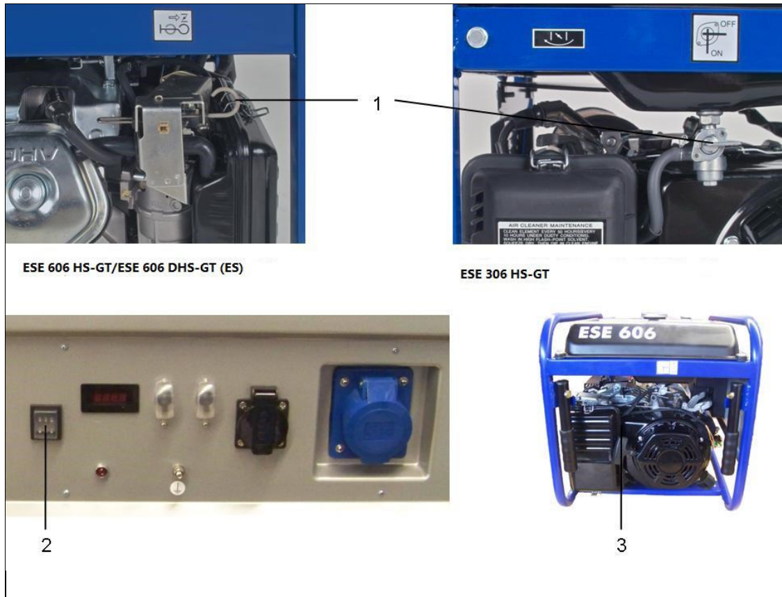
Abb. 4.2: Motor starten
