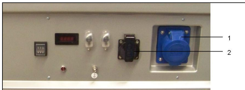
Abb. 4.3: Verbraucher anschließen
