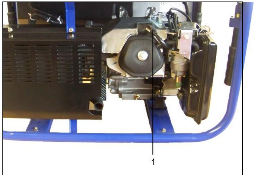
Abb. 4.7: Zündkerzenstecker abziehen
